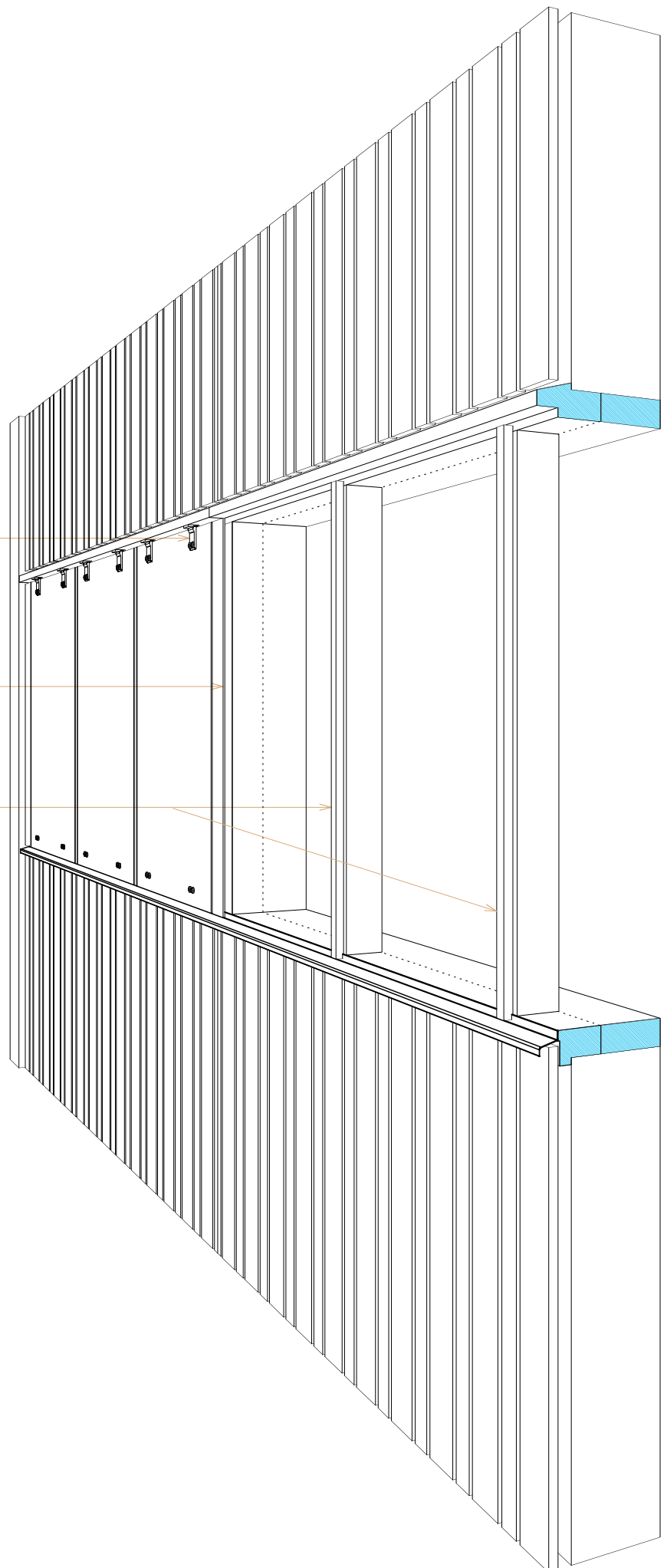
3D weergave kozijn samenstelling voorgevel
